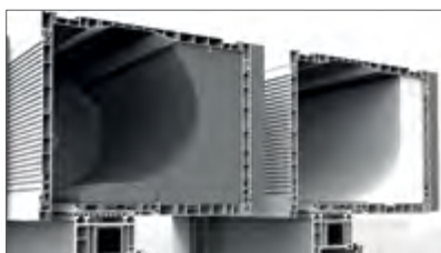
Verschiedene Isolationsarten des Boxes für die optimale Anpassung an die klimatischen Bedingungen (Version aus Neopor® oder Styropor®)
