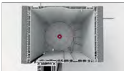
Doppellagersitz für eine optimale Ausrichtung der Panzerwelle in der Wickelfunktion
