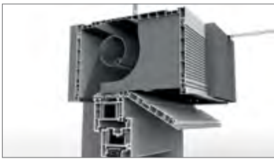
Tiefer Gehäusebox mit Revisionsabdeckung von unten (ganze Bebauung möglich)
